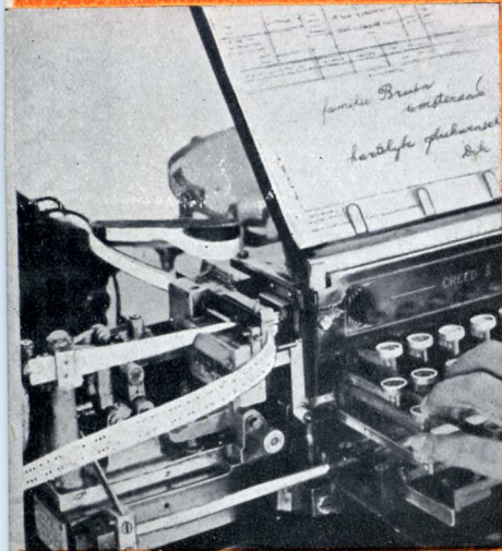
AUTOMATISCH TELEGRAAFTOESTEL.
