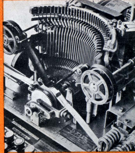
AUTOMATISCH SCHRIJFONTVANGTOESTEL.
