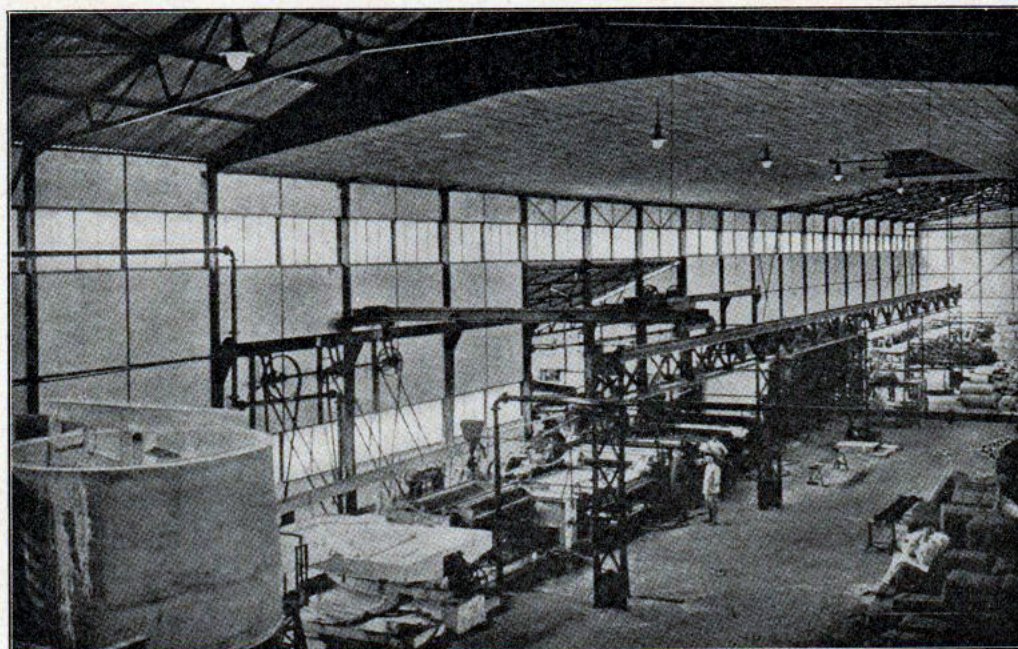
436. PAPIERFABRIEK TE PADELARANG VAN BINNEN.
