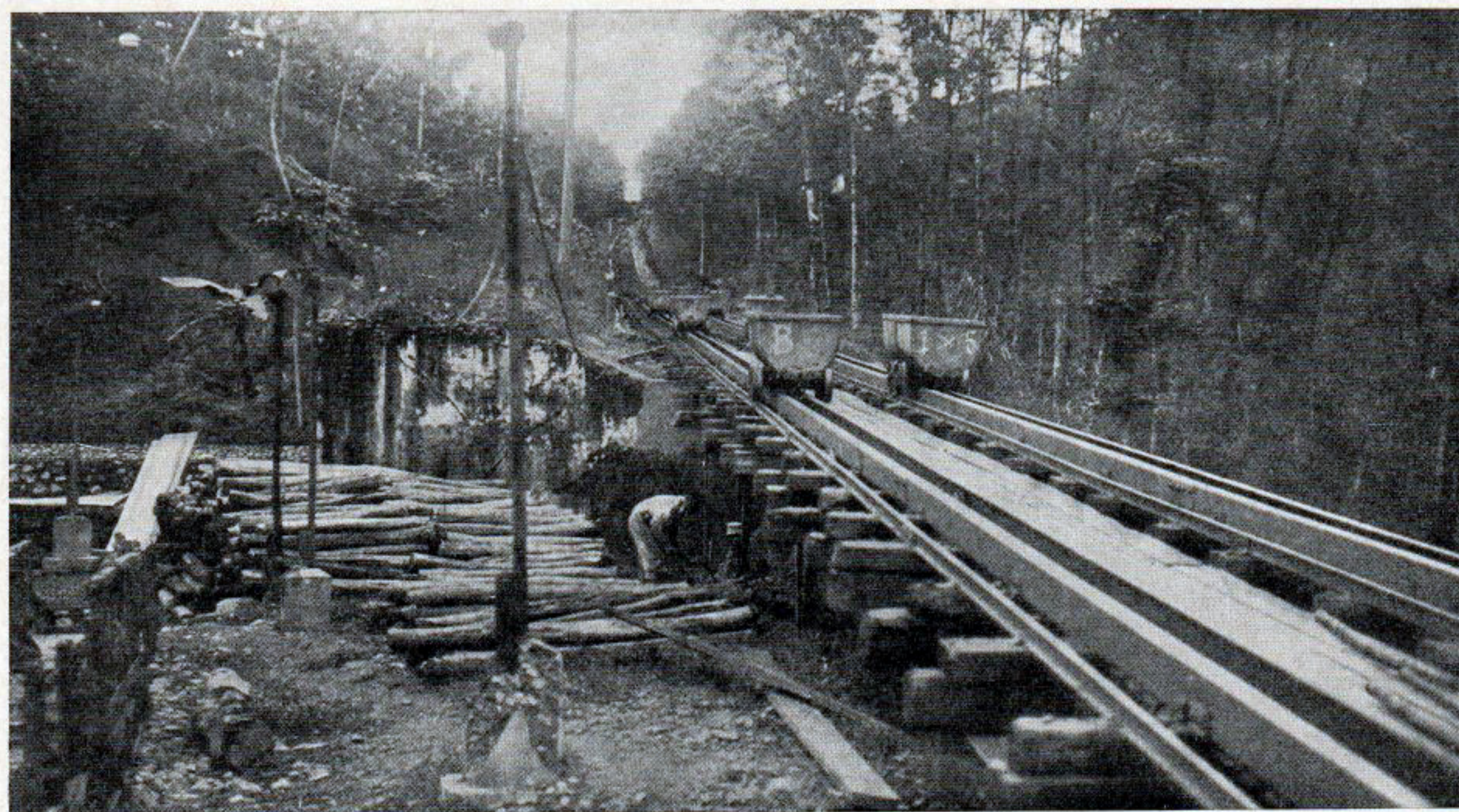
467. ELECTRISCH MIJNSPOOR BIJ SAWAHLOENTO.
