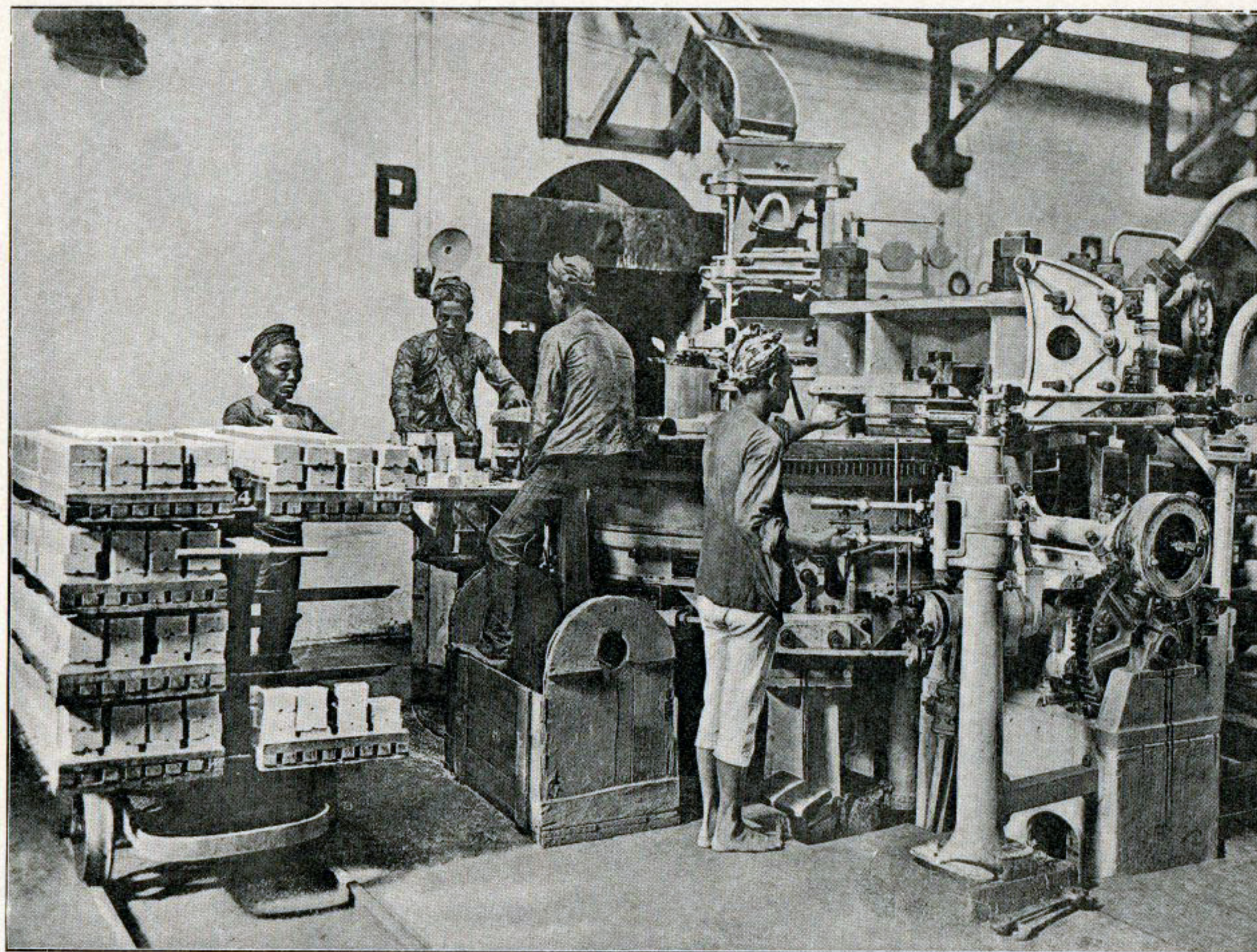
476. AAN EEN BRIKETPERS IN EEN FABRIEK OP MADOERA.
